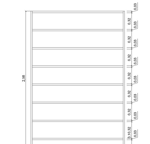
VISTA A- FRONTAL medidas em metros
